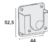
Soporte
